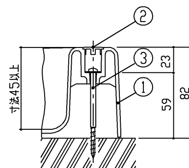
固定部詳細(1/3)
